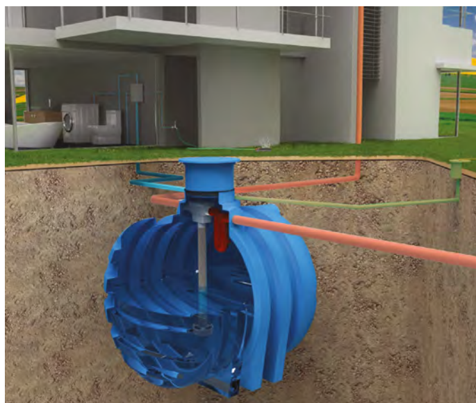
NEPTUN instalovaný s přítokovým setem
